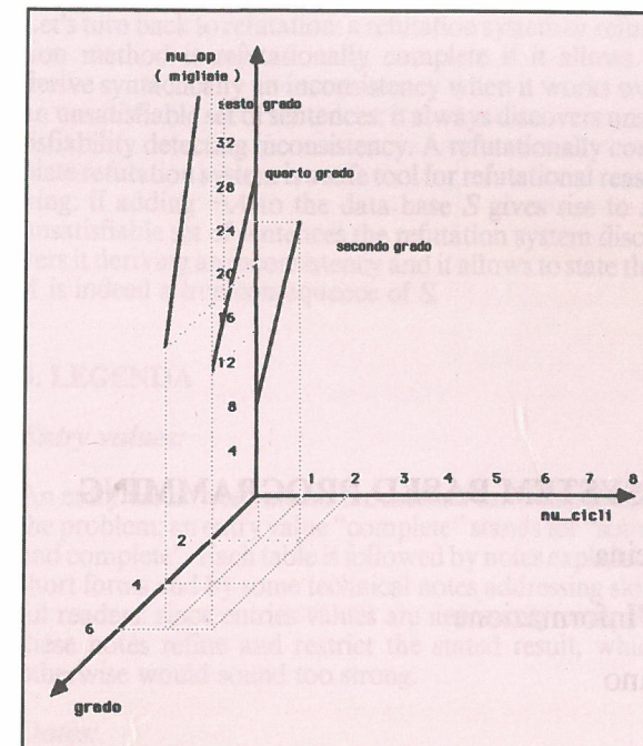
Fig. 5 Relazione tra il numero di operazioni, numero di cicli e il grado del polinomio.
