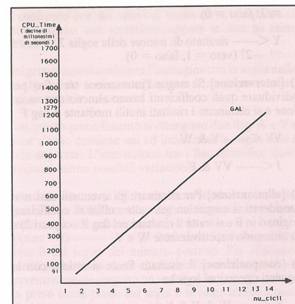
Fig. 4 Ipotesi: 10 MHz programmi GAL (valori teorici)
