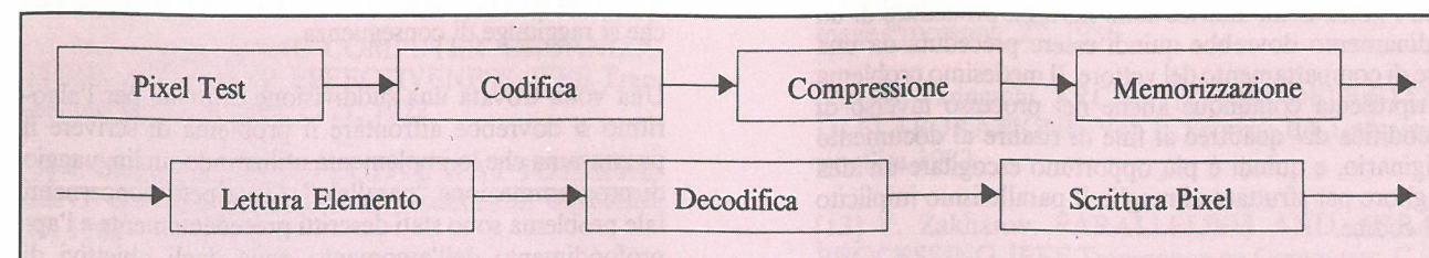
Fig. 7 Soluzione "pipeline" per l'algoritmo.
