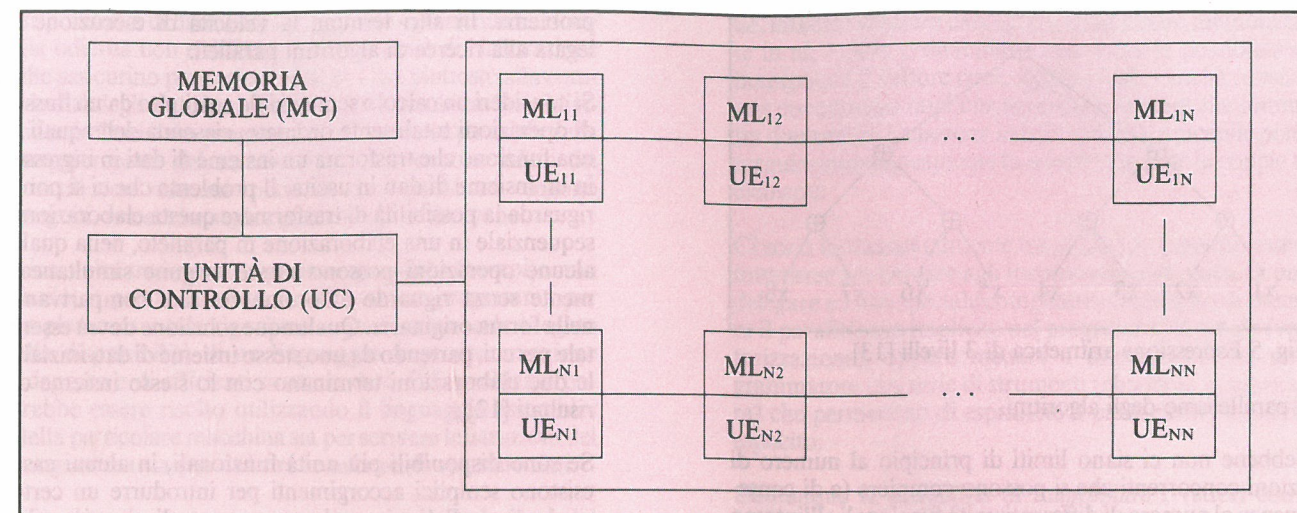
Fig. 4 Schema di un "array processor" (da [12]) (ML = Memoria Locale; UE = Unità di Elaborazione).
