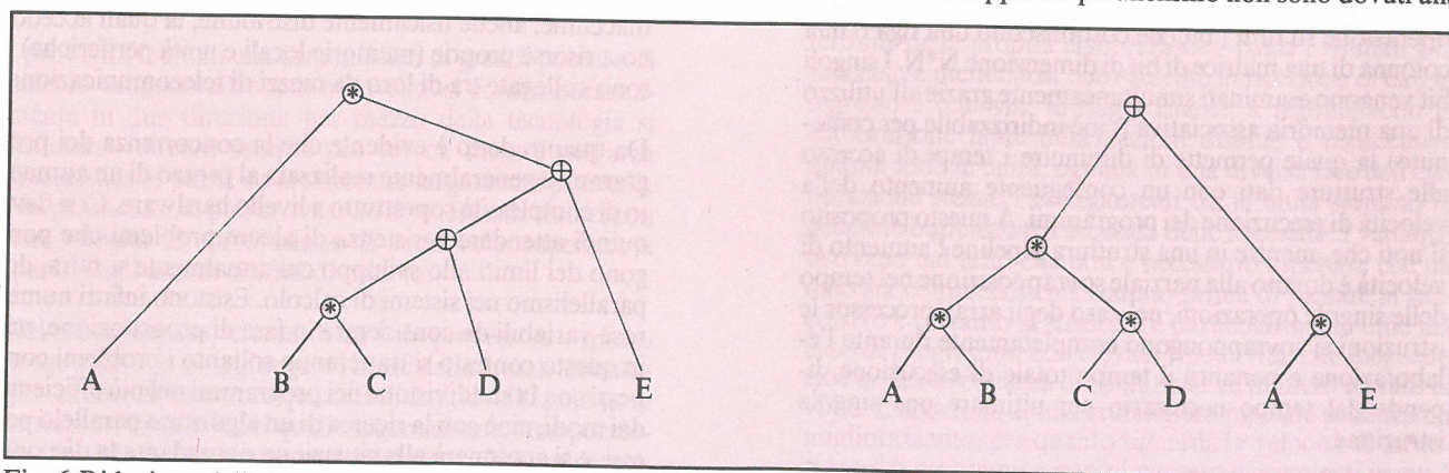
Fig. 6 Riduzione dell'altezza dell'albero mediante l'applicazione della proprietà distributiva all'espressione A(BCD+E) [13].
