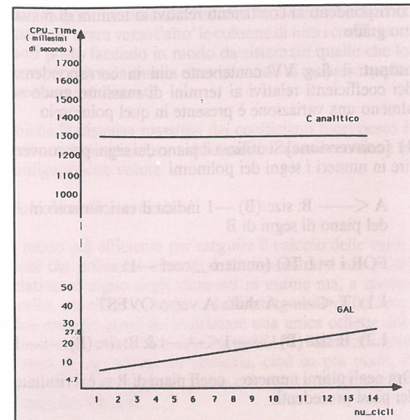
Fig. 3 Ipotesi: 4.77 MHz programmi C - 4.77 MHz programma GAL (valori teorici)
