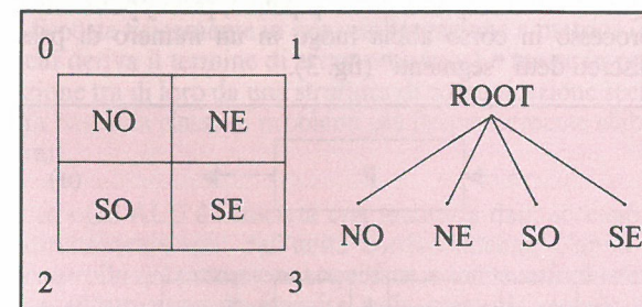
Fig. 1 Divisione dello spazio bidimensionale in quadranti e relativa rappresentazione del quadtree.
