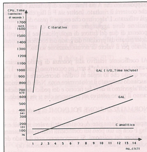
Fig. 2 Ipotesi 4.77 MHz programmi C - 30 KHz programma GAL.
